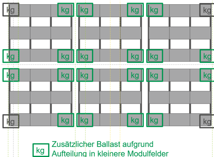
Abbildung 2: Aufteilung eines großen Modulfeldes in drei kleinere Modulfelder
