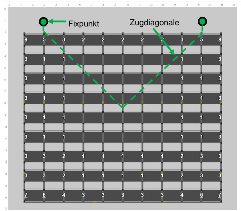
Abbildung 5: Ballastplan mit Angabe der Ballastierung in Anzahl Steine (à 10kg)
