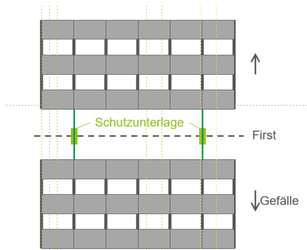
Abbildung 1: Kopplung zweier Felder mit unterschiedlichem Gefälle
